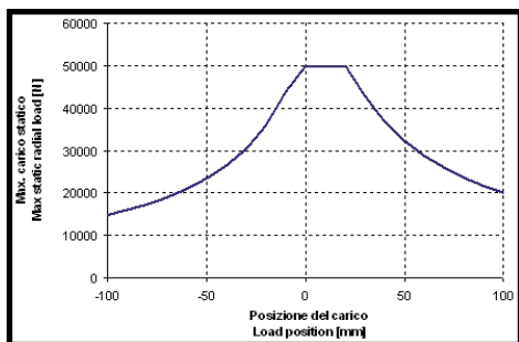
La posizione "0" coincide con la flangia ruota Position "0" is coincident with wheel mounting
